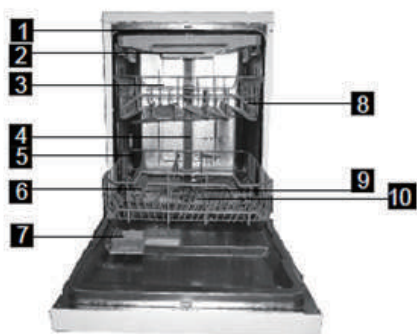
正視圖
