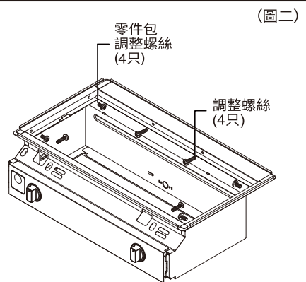
固定本體
