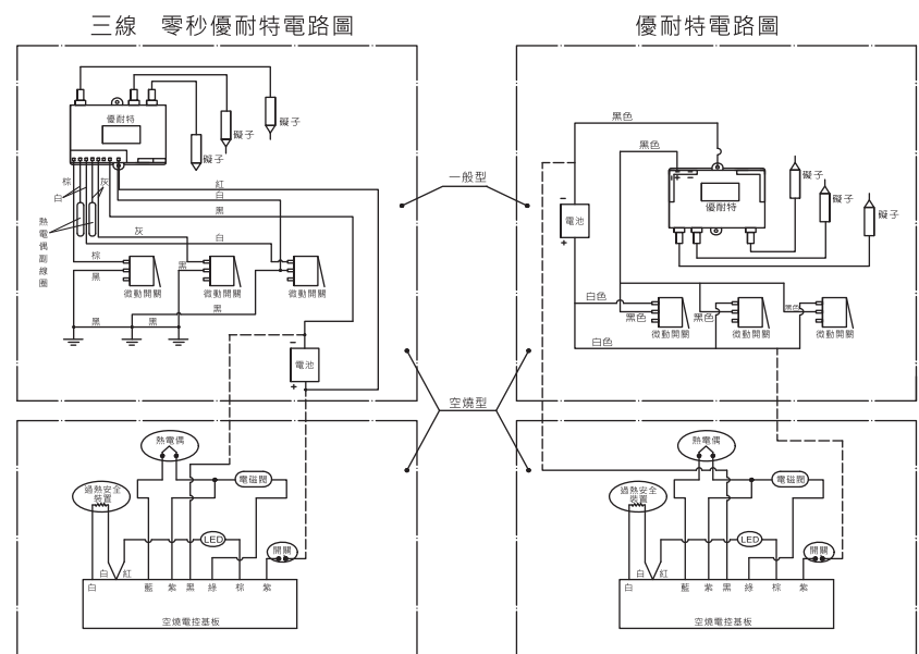
優耐特電路圖
