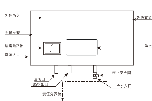
■ 橫掛式TE-2120W(6KW)加侖配管圖
