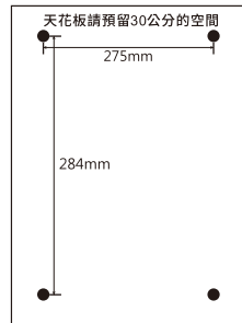
2.鑽孔 \phi 10 \times 4 (2分半膨脹螺絲)
