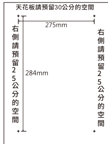
1.捲尺測量鑽孔位置尺寸圖(請留意水平)
