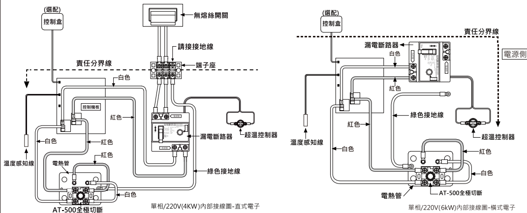
單相/220V(4kW)內部接線圖-直式電子
