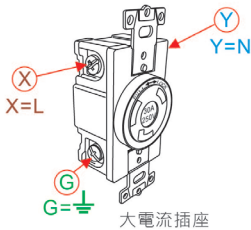
大電流插座&插頭配線示意圖
