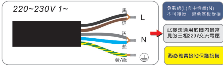
大電流插座&插頭配線示意圖
